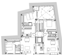
PLANTA CUARTO PISO
