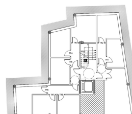
PLANTA QUINTO PISO
