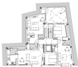
PLANTA TERCER PISO
