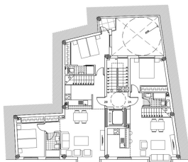
PLANTA CUARTO PISO
