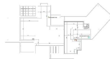
PLANTA CUBIERTA
