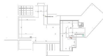
PLANTA CUBIERTA
