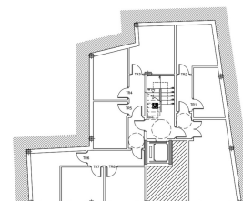
PLANTA SEMISOTANO
